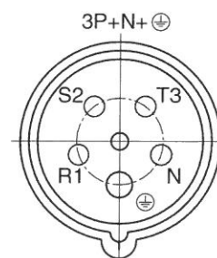
Kobl. 400V (5 pins)
